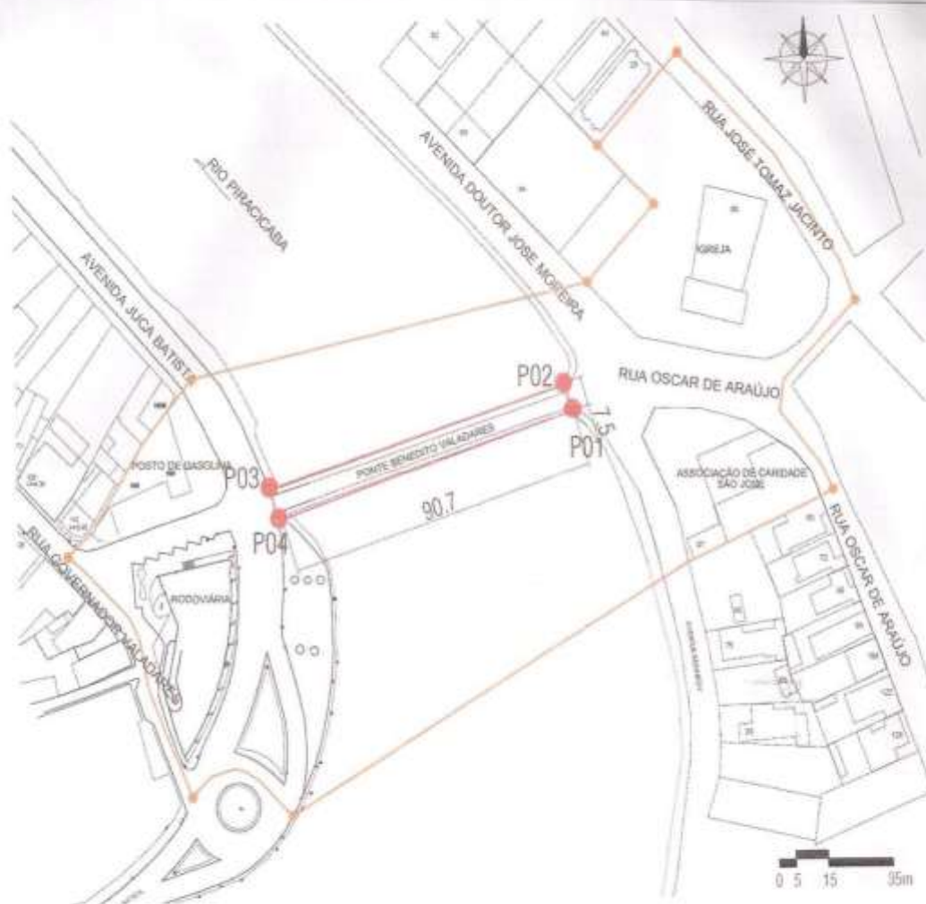
Figura 01 - Delimitação do perímetro de tombamento da Ponte Benedito Valadares Área tombada: 680, 25 m 2 – Área construída: 680, 25 m 2 Elaboração: Fabiane Cristine Fonseca – Setembro/2016.
