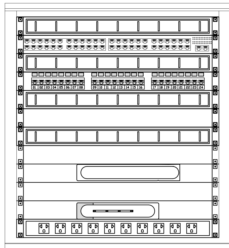
RACK 32U - EQUIPAMENTOS INTERNOS SEM ESCALA
