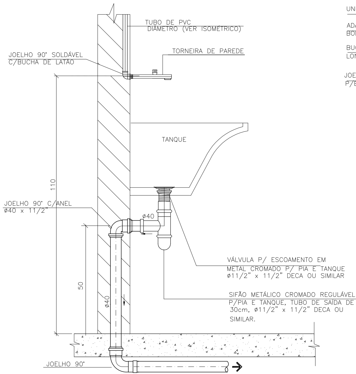
DETALHE – INSTALAÇÃO DO TANQUE
