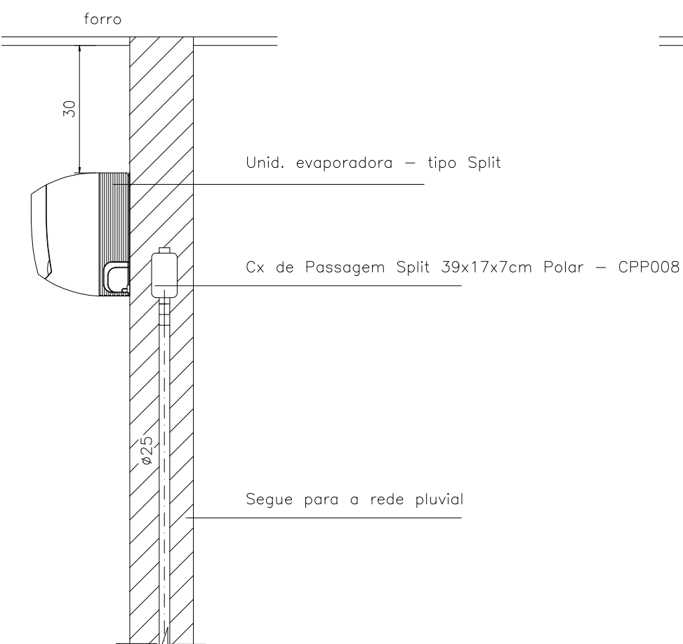
VISTA LATERAL
