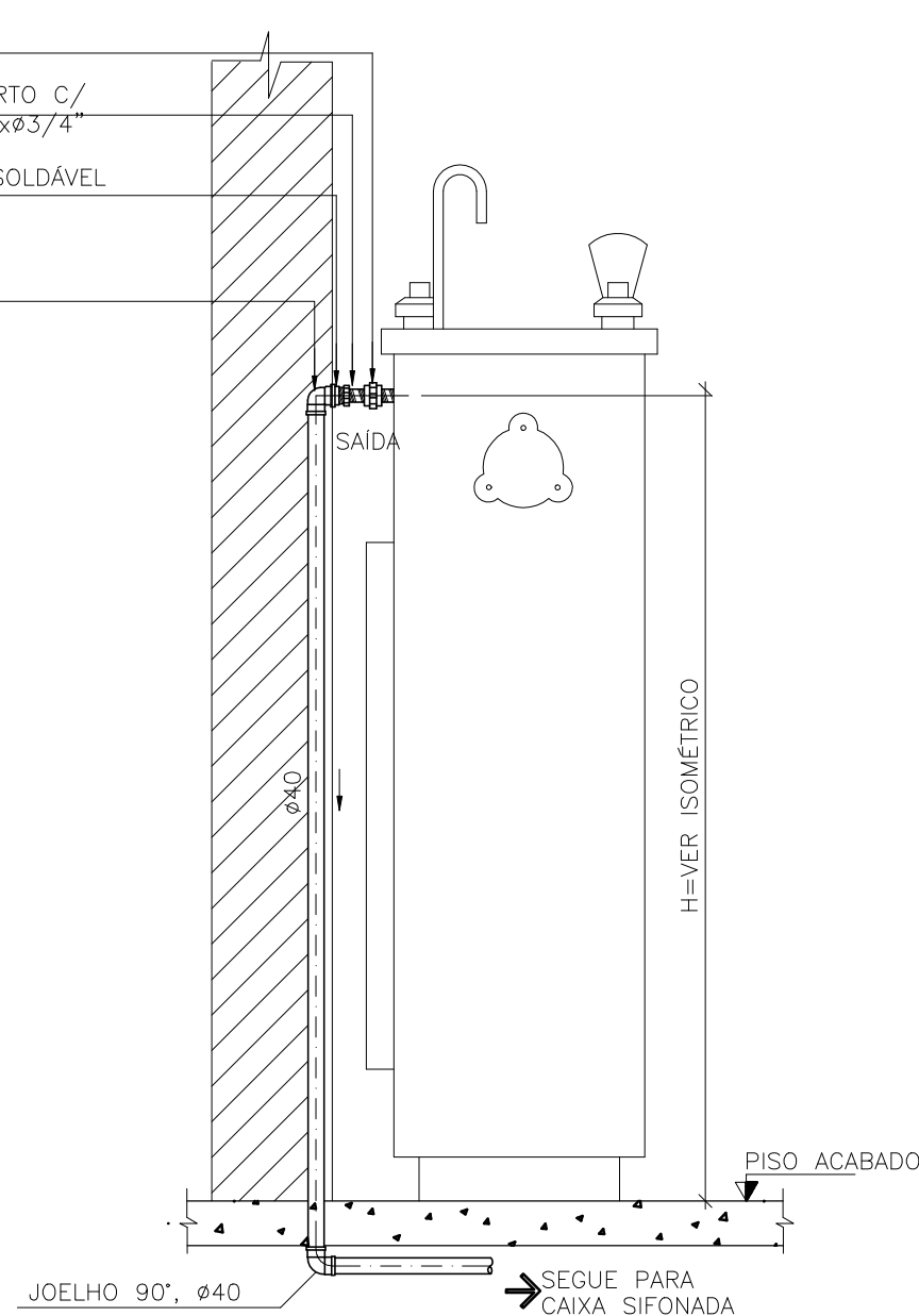
VISTA LATERAL
