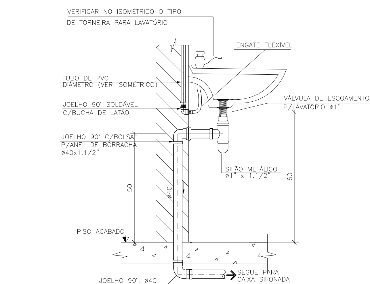
DETALHE – INSTALAÇÃO DO LAVATÓRIO
