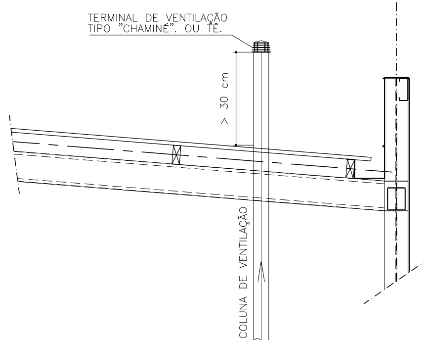
DETALHE – TORRE DE VENTILAÇÃO
