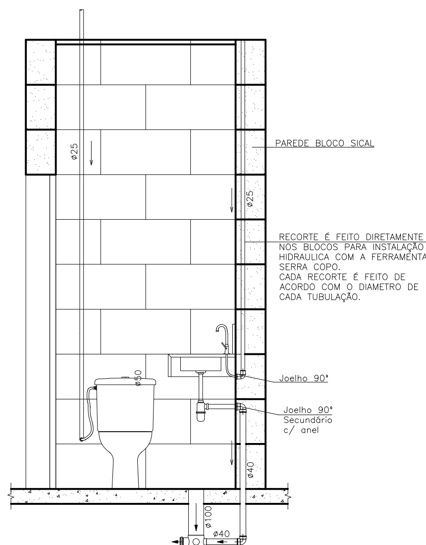
DETALHE – INSTALAÇÃO EM BLOCO SICAL
