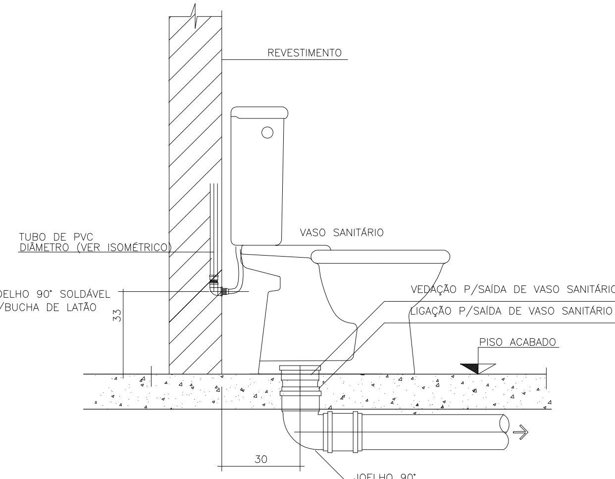
DETALHE – LIGAÇÃO DO VASO SANITÁRIO
