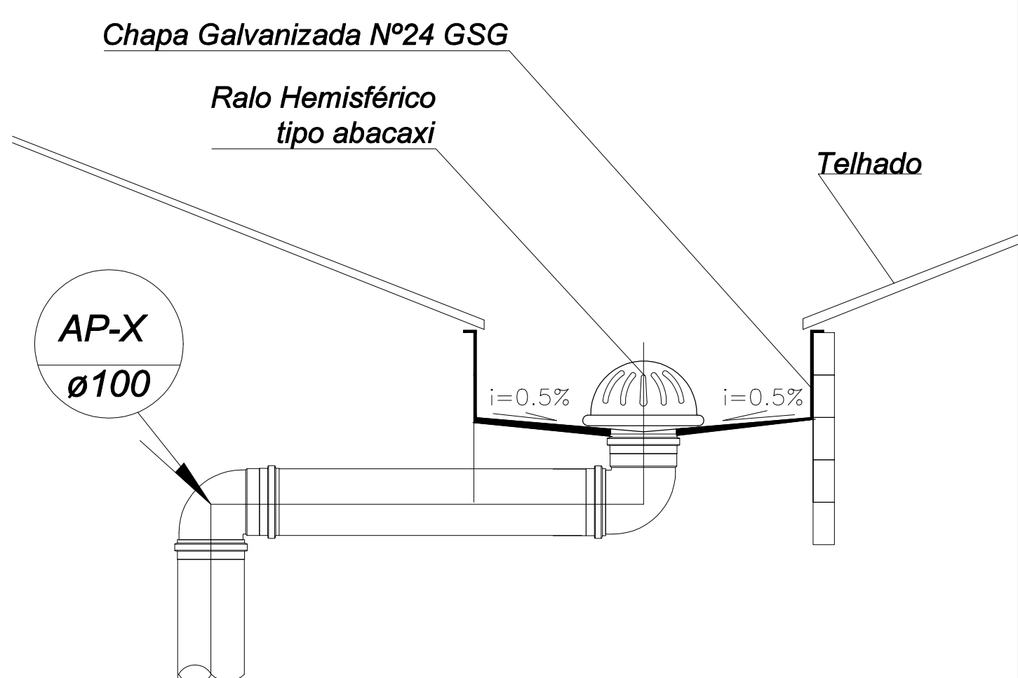
DETALHE – CALHA
