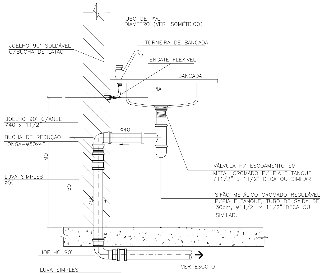
DETALHE – INSTALAÇÃO DE PIA
