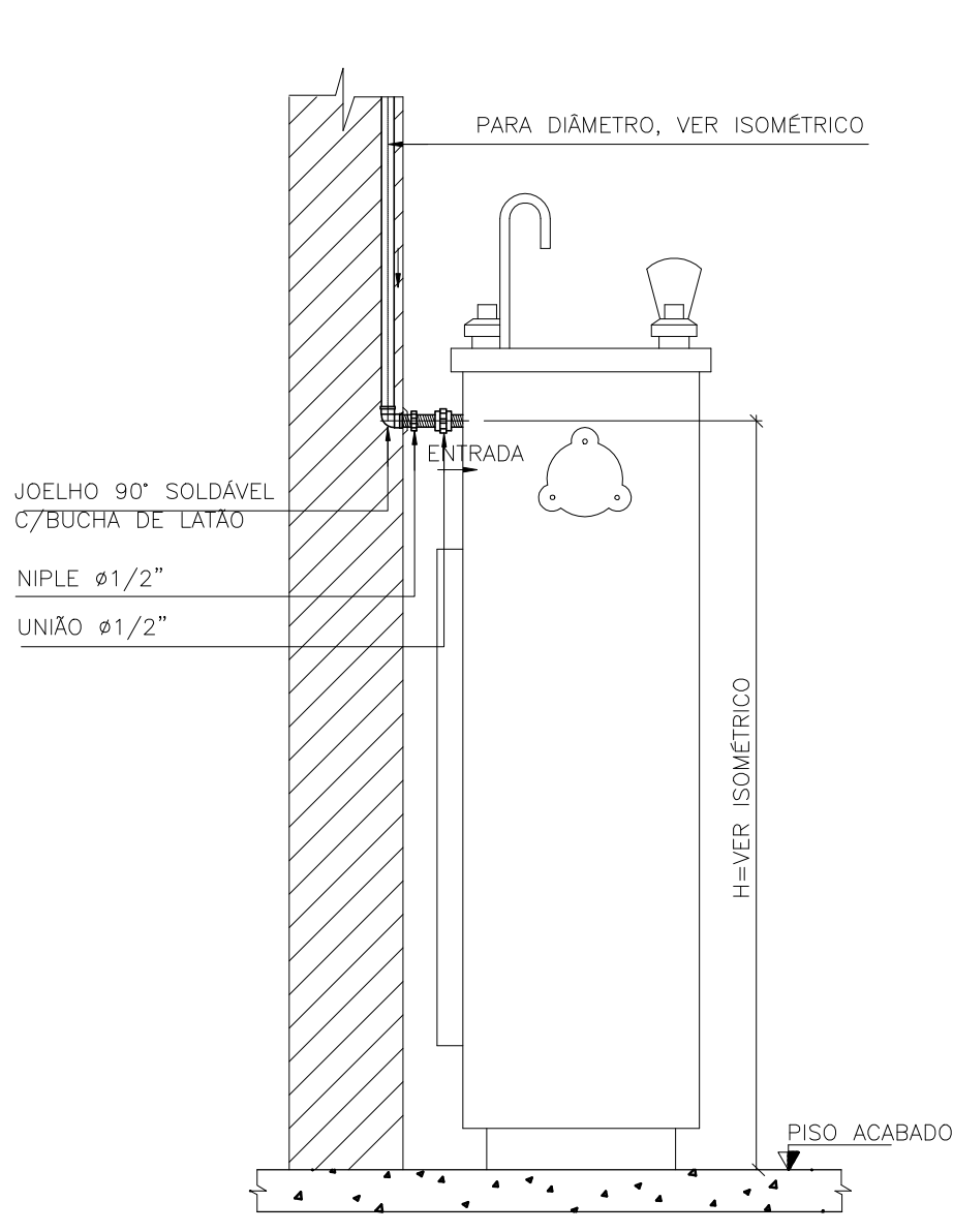
VISTA LATERAL
