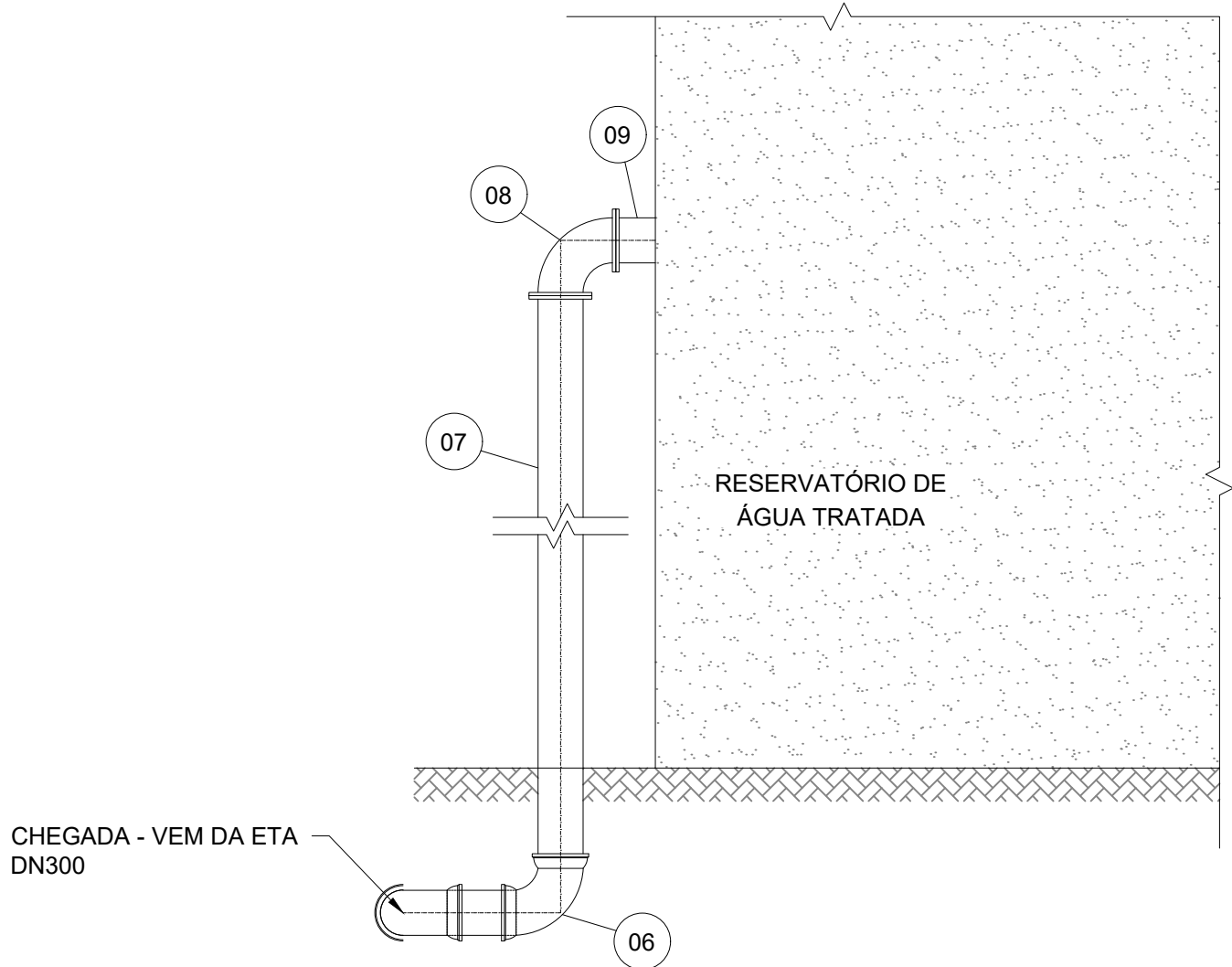
DETALHE DA CHEGADA NO RESERVATÓRIO ESC.: 1/50
