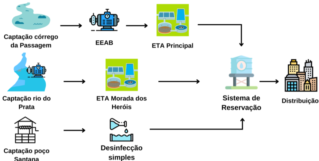
Figura 1 - Fluxograma do Sistema de Abastecimento de Água existente
