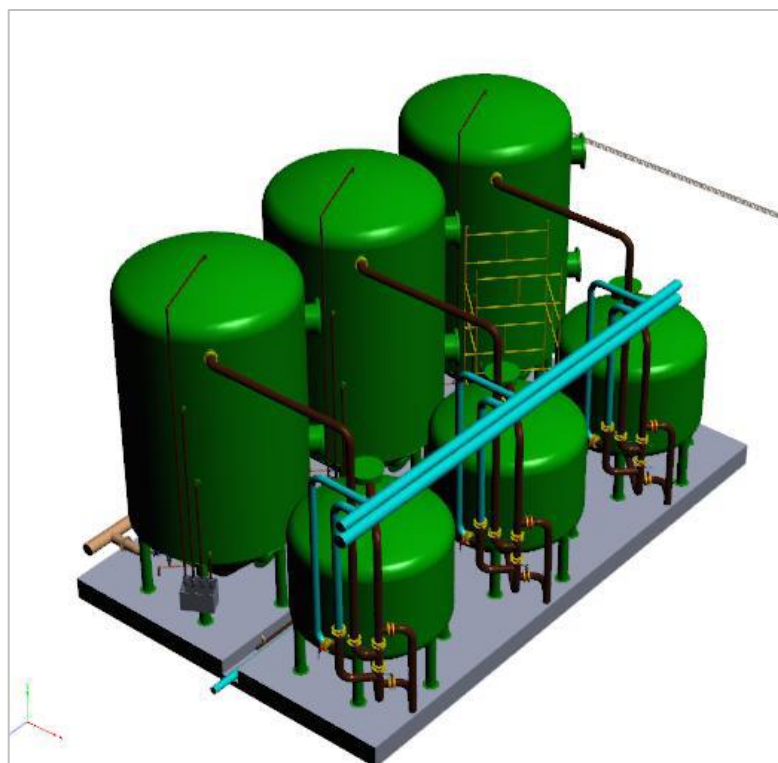
Figura 9 – Módulos com floco decantador e filtro
