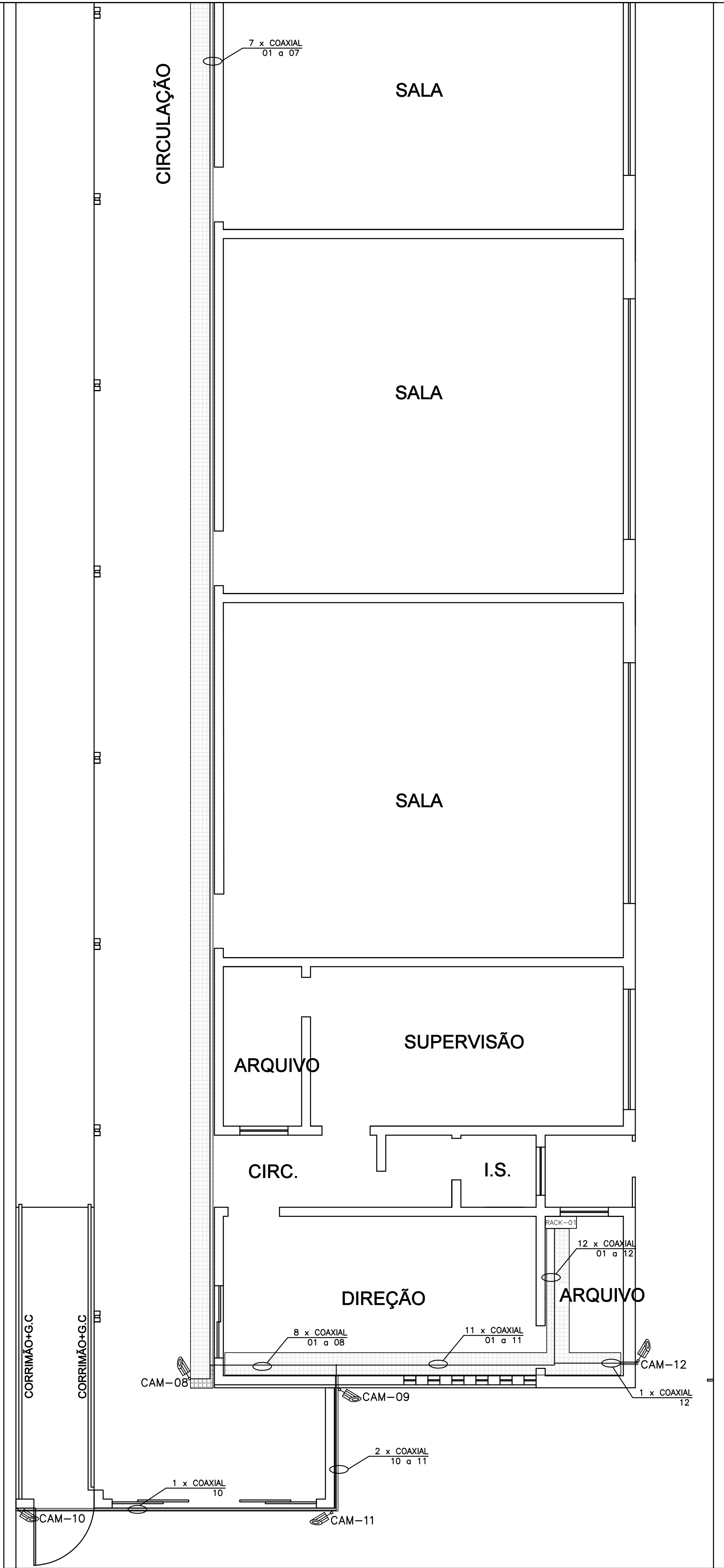
CIRCUITO DE CÂMERAS ESCALA 1/50
