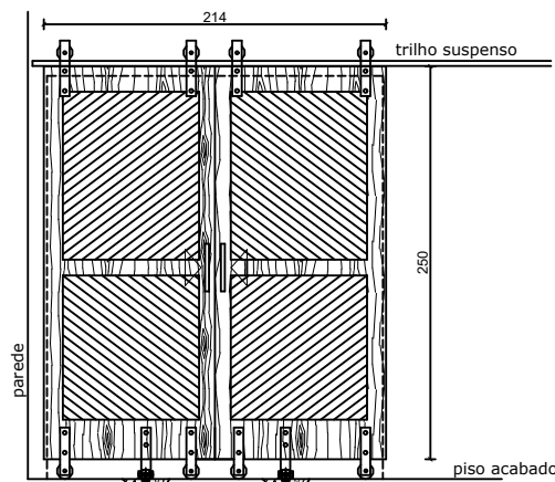
VISTA TRAS. PORTA DE CORRER (SALAS, BL. 1) Esc: 1/40
