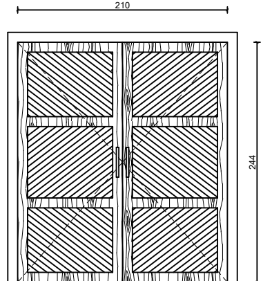
VISTA PORTA (SALA 4) Esc: 1/40
