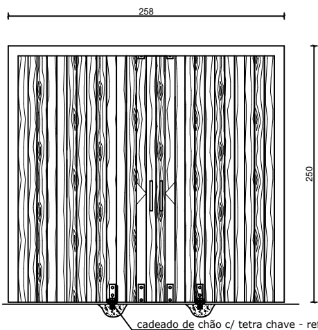
VISTA FRONT. PORTA DE CORRER (SALAS BL. 2) Esc: 1/40
