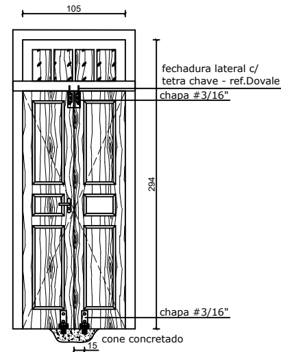
VISTA TRAS. PORTA BRINQUEDOTECA Esc: 1/40
