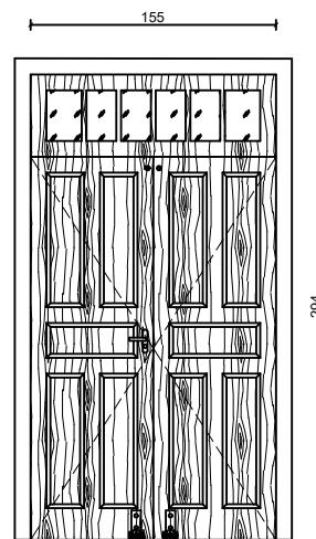
VISTA PORTA BIBLIOTECA Esc: 1/40
