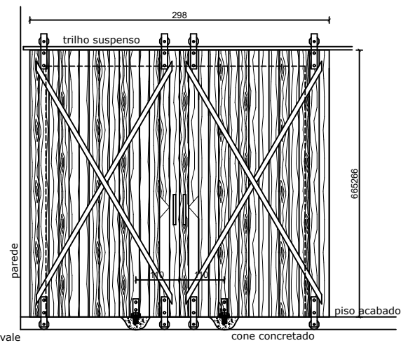
VISTA TRAS. PORTA DE CORRER (SALAS BL. 2) Esc: 1/40
