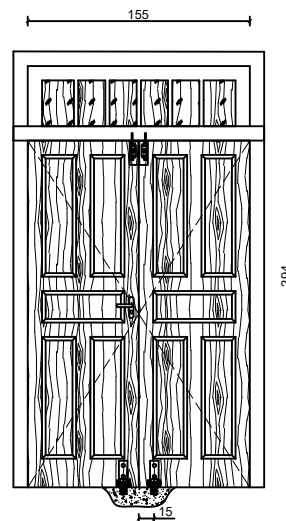
VISTA TRAS. PORTA BIBLIOTECA Esc: 1/40
