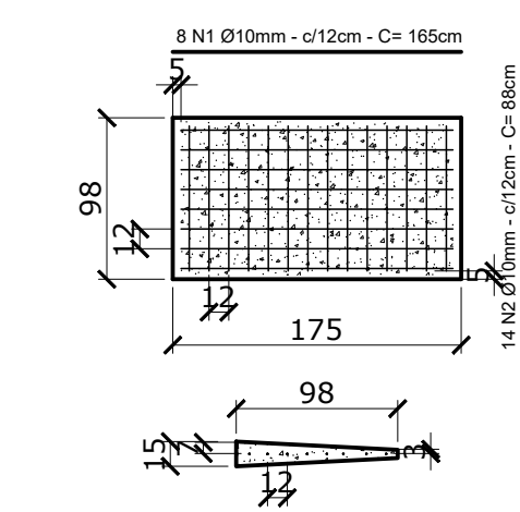
ARMAÇÃO DA LAJE
