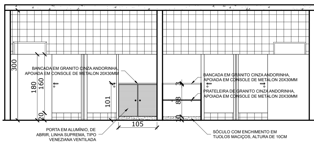
CORTE C-C
