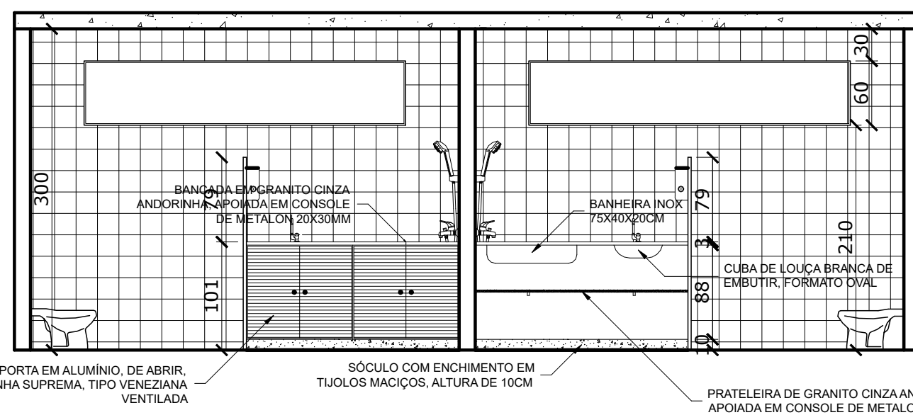
CORTE D-D
