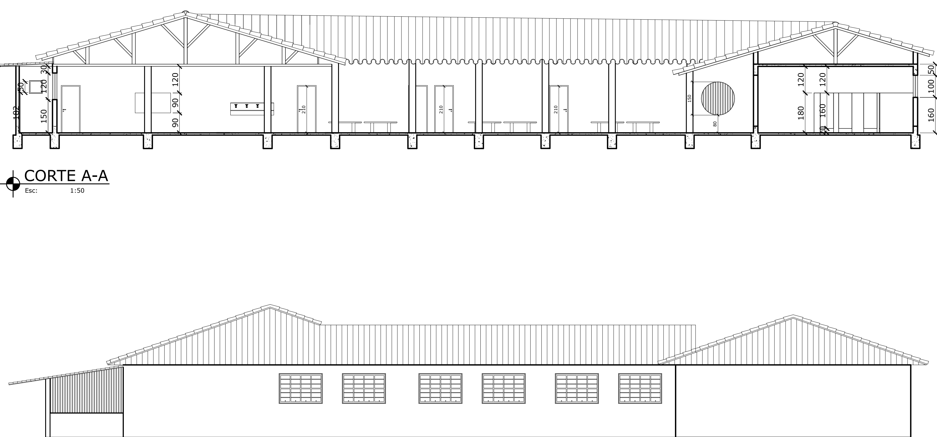
FACHADA
