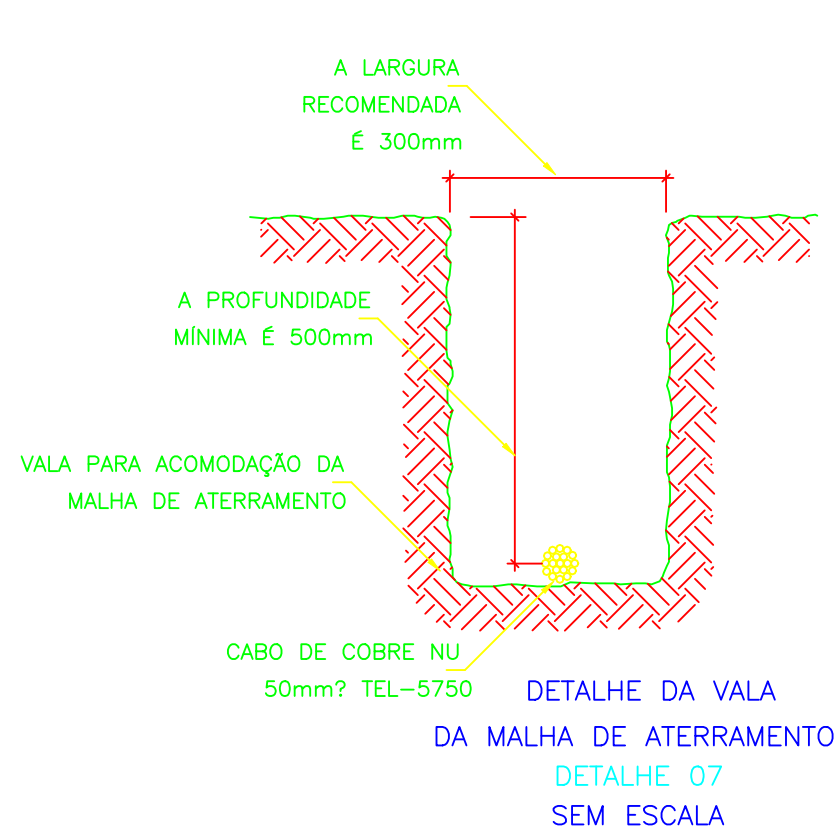
DIAGRAMA DE ATERRAMENTO – SEDE
