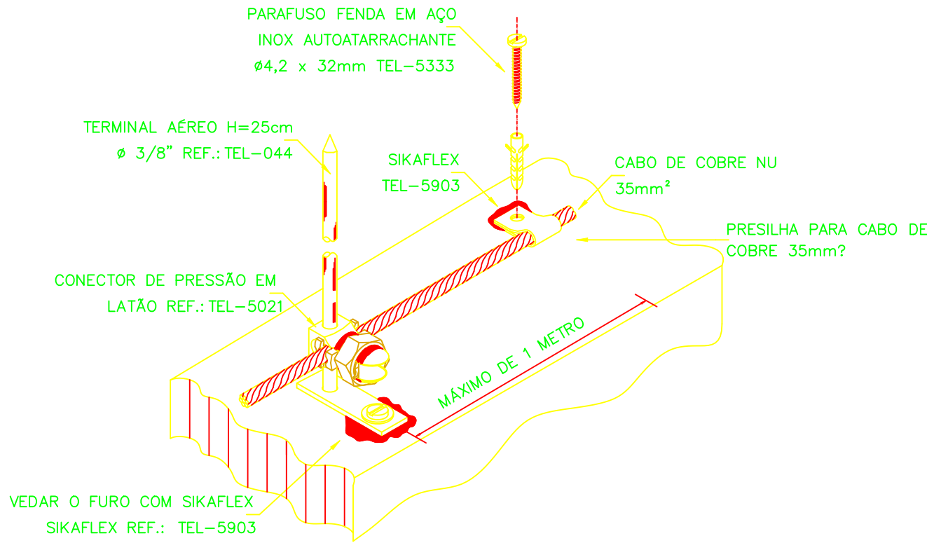
DETALHE DE FIXAÇÃO DO CABO DE COBRE E TERMINAL AÉREO NA PLATIBANDA DETALHE 04 SEM ESCALA
