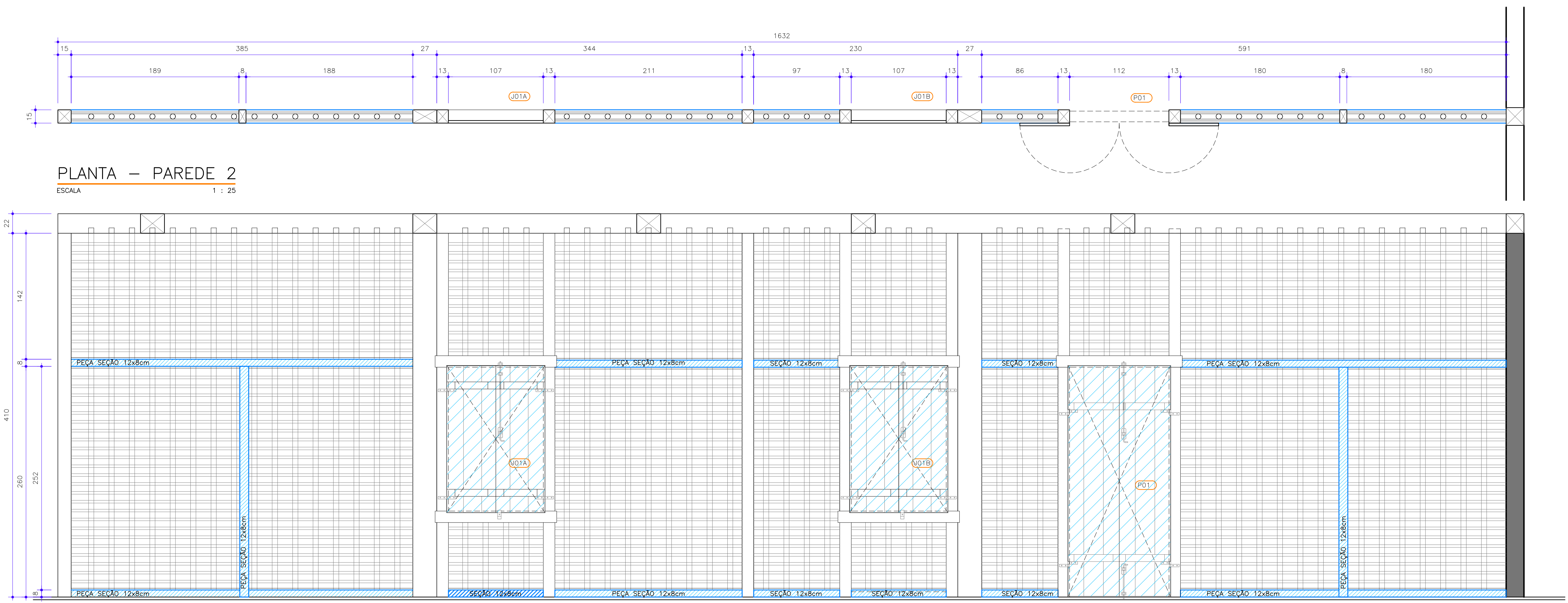
VISTA B – ARMAÇÃO PAU-A-PIQUE/ PAREDE 2 ESCALA 1 : 25
