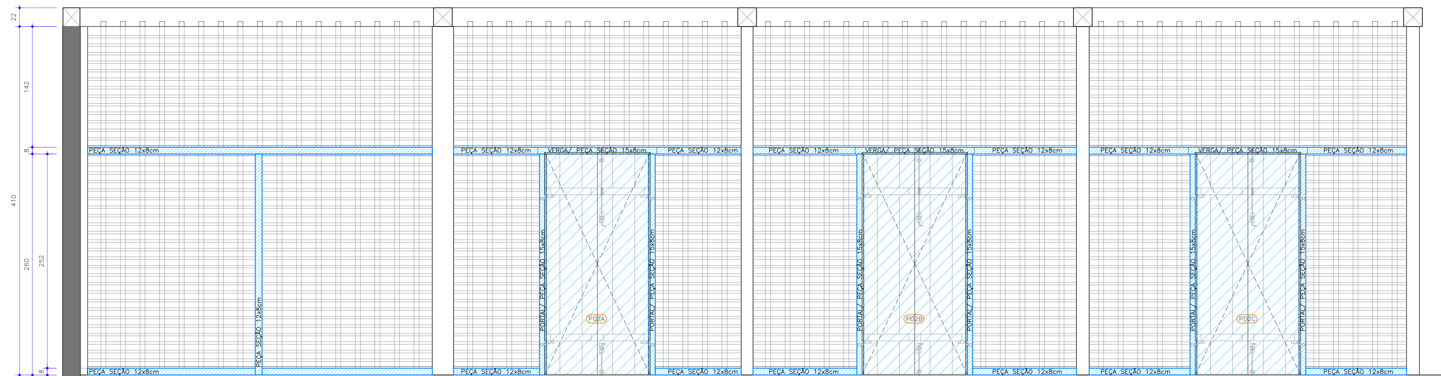
NOTA: AS REGIÕES HACHURADAS EM AZUL CORRESPONDEM ÀS NOVAS PEÇAS A SEREM INSTALADAS
