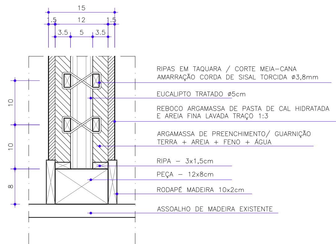
DETALHE 03 ESCALA 1 : 5
