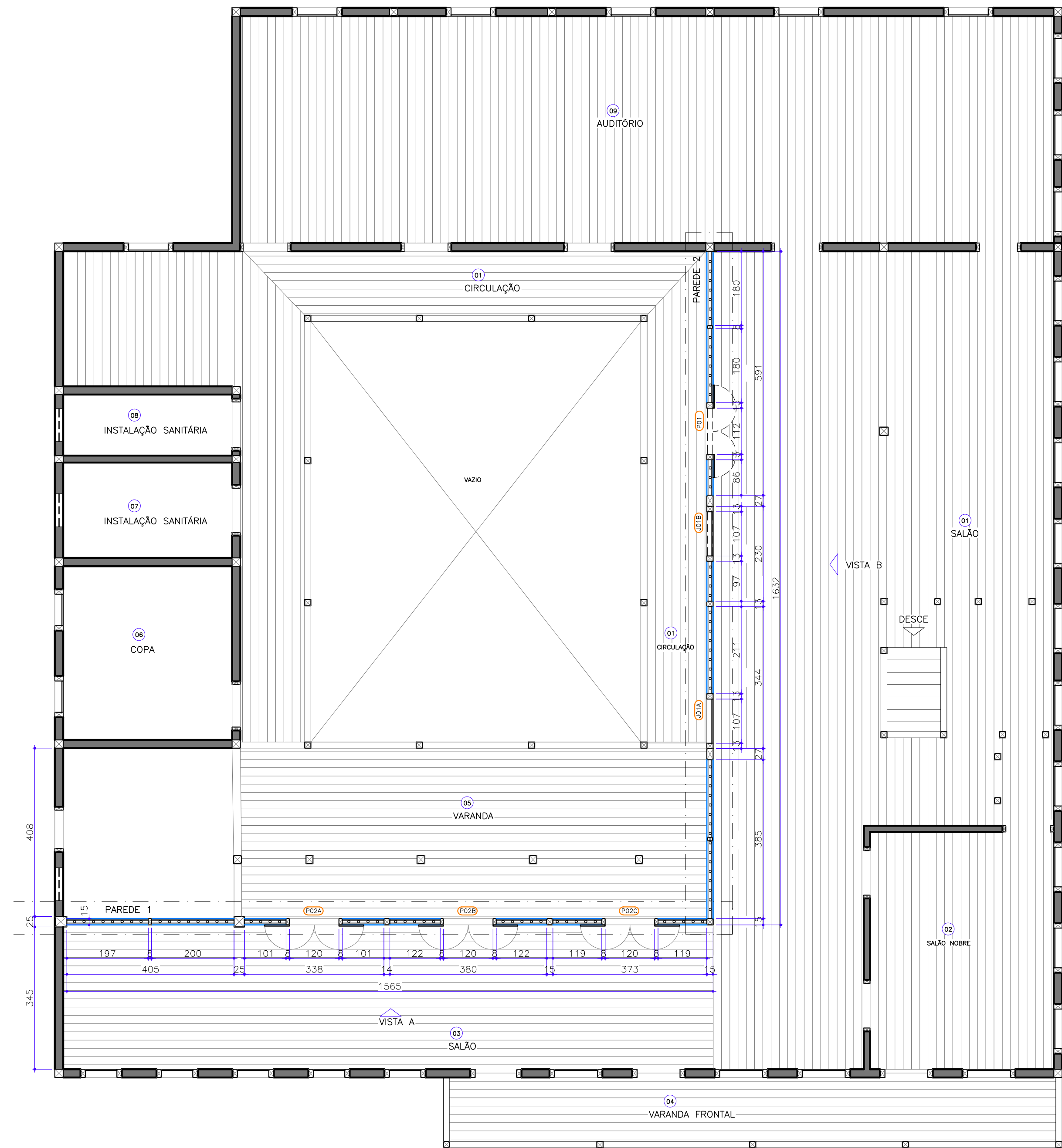
PLANTA PAVIMENTO SUPERIOR ESCALA 1 : 75
