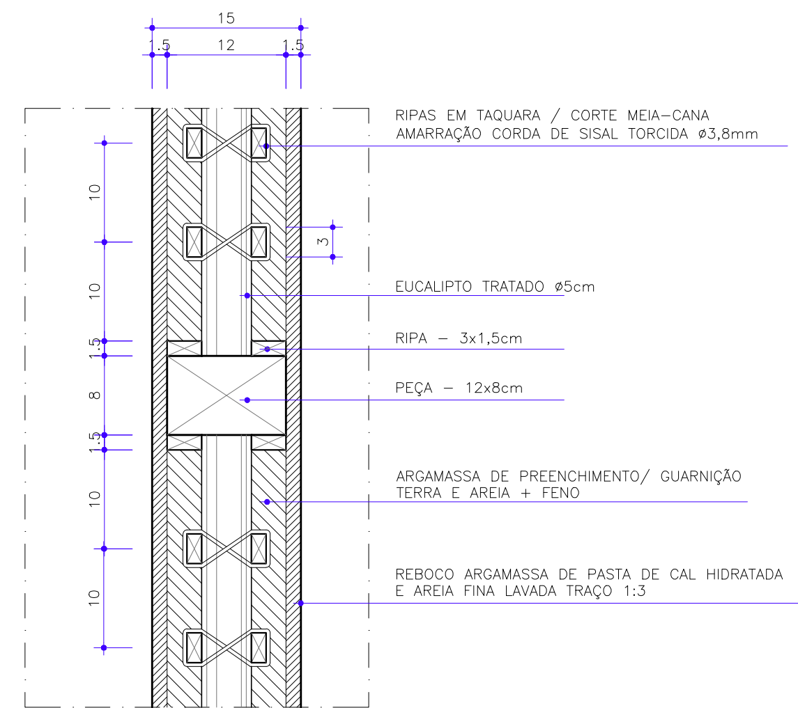
DETALHE 02 ESCALA 1 : 5
