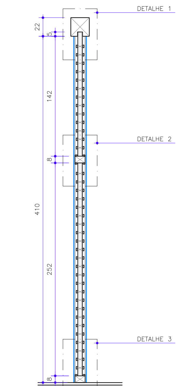
SEÇÃO VERTICAL TIPO PAREDE PAU-A-PIQUE ESCALA 1 : 25
