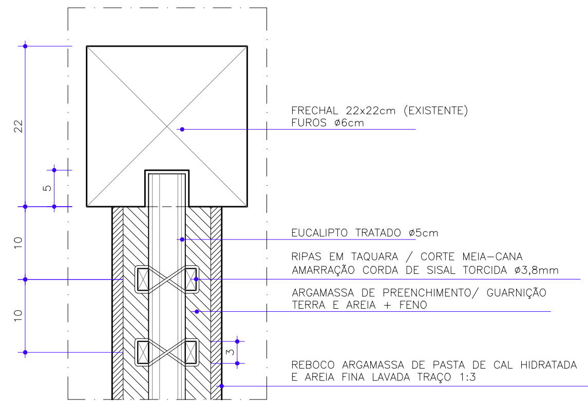
DETALHE 01 ESCALA 1 : 5
