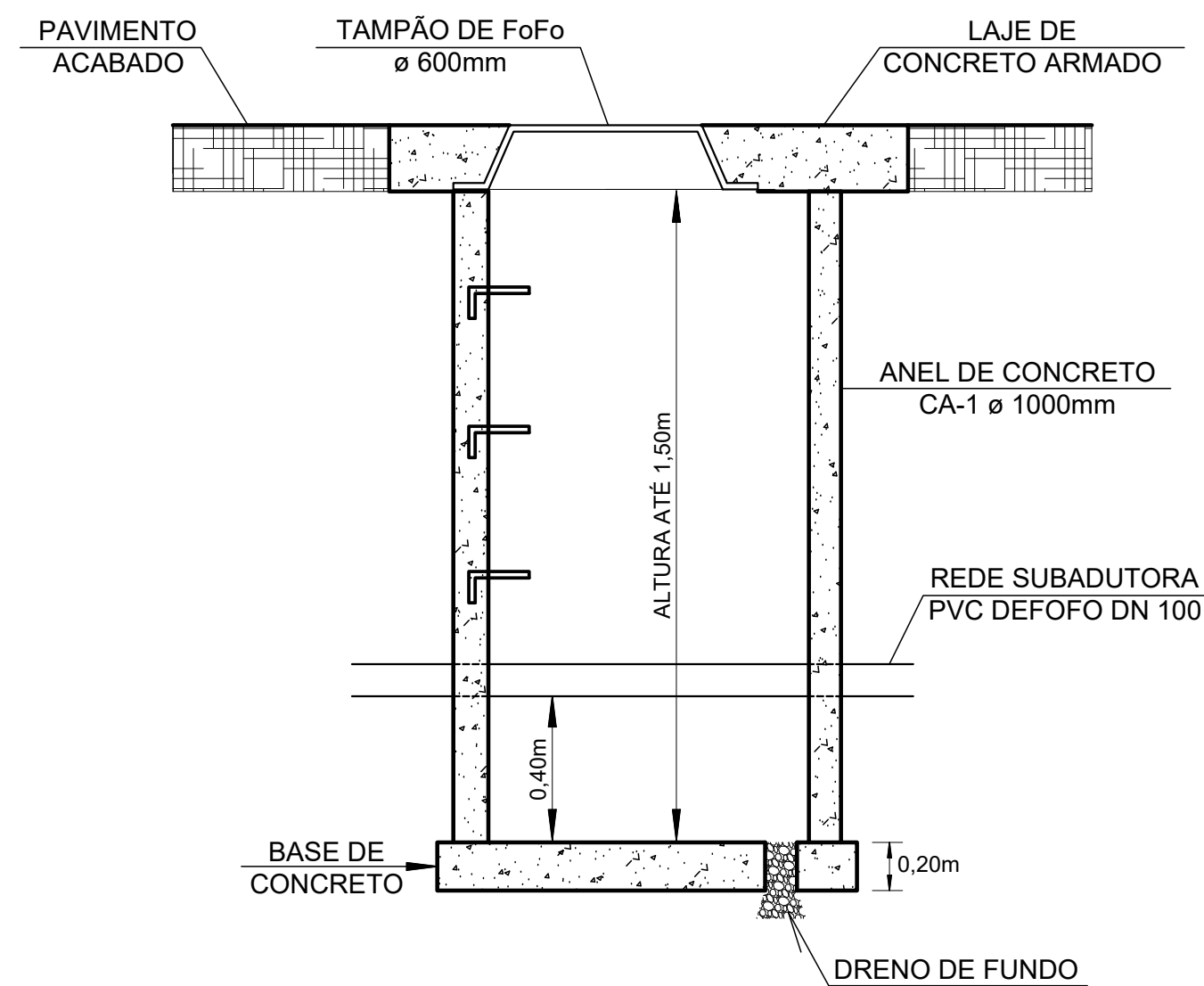
CORTE AA
