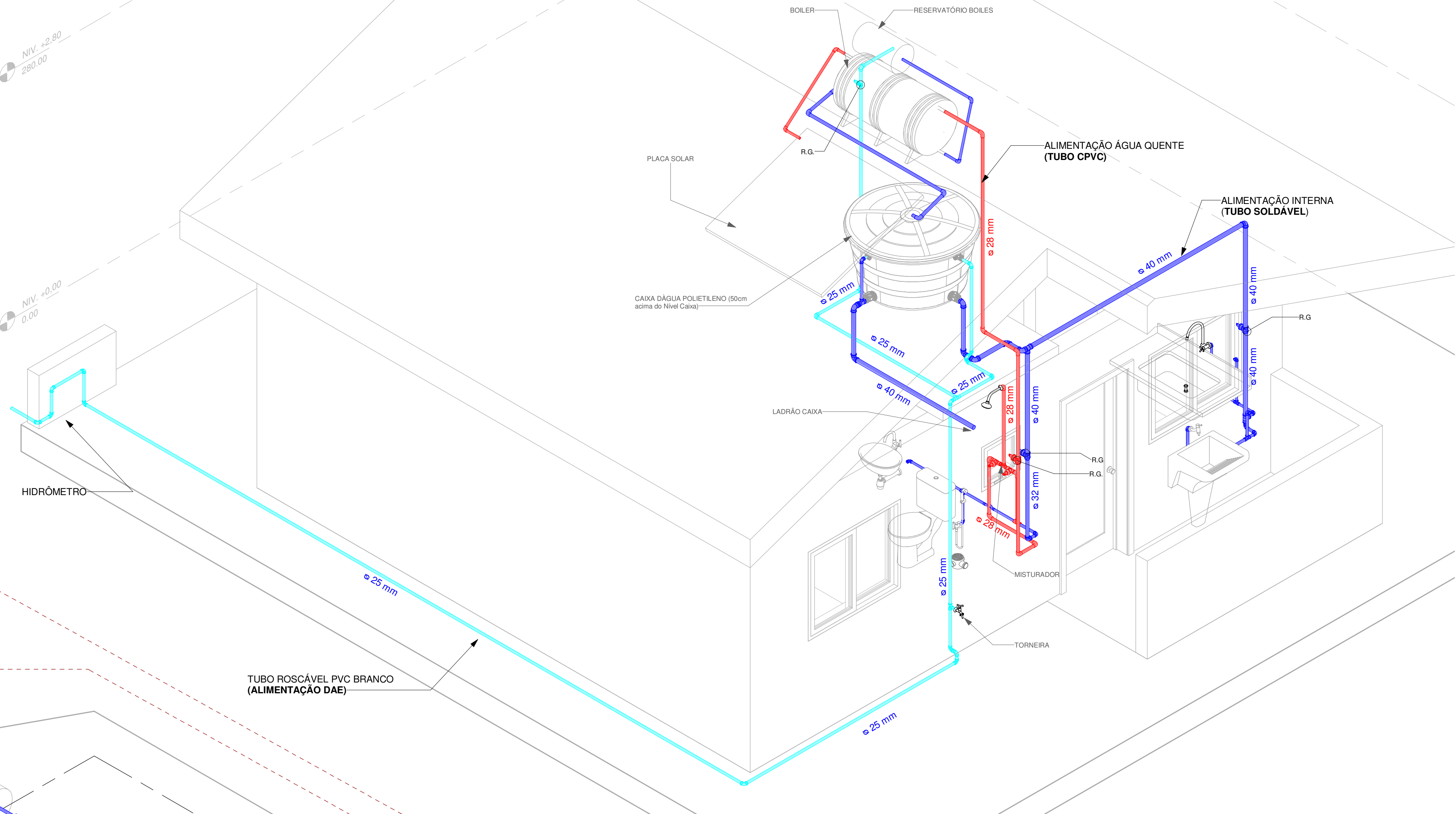
1 Isométrico AF/AQ (Geral)
