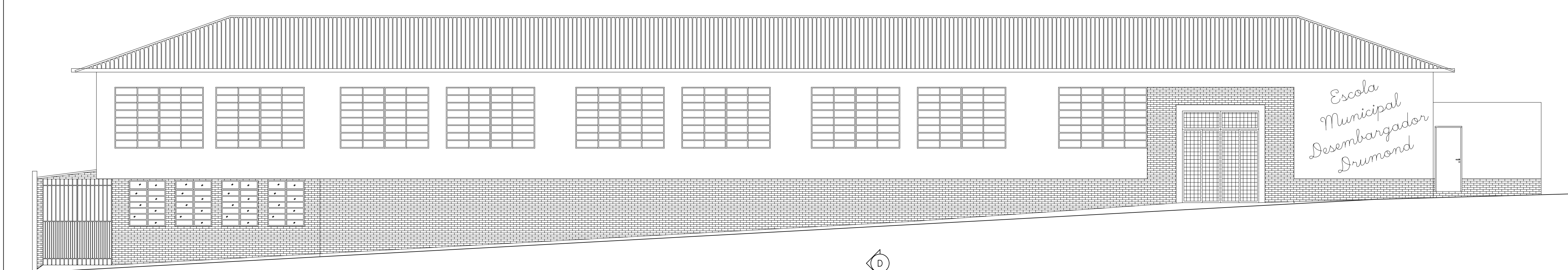
FACHADA Esc: 1:75
