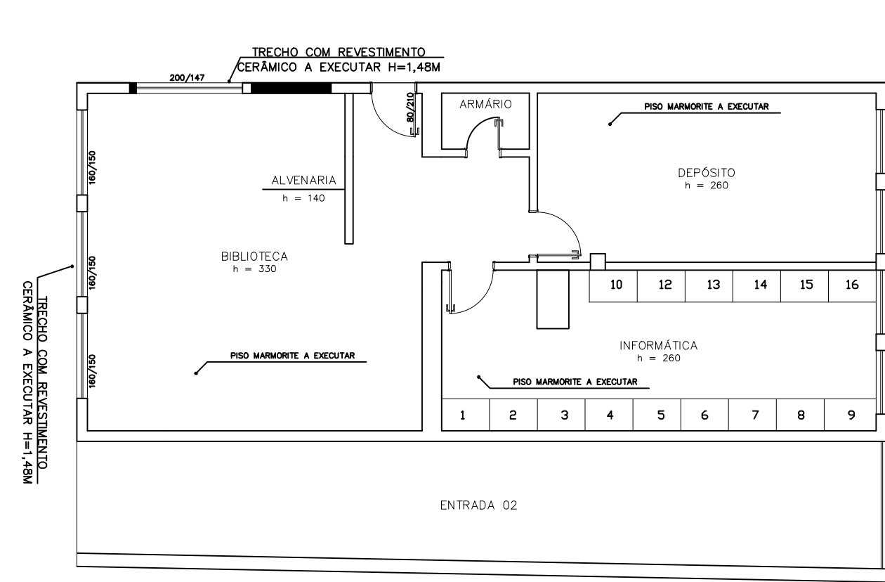
PLANTA BAIXA - BIBLIOTECA Esc: 1:100
