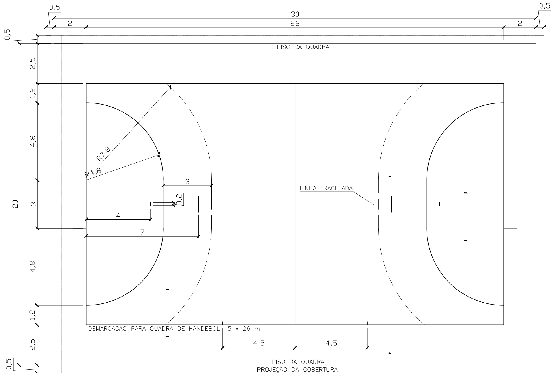
ANEXO 3: DEMARCAÇÃO DE LINHAS DA QUADRA DE HANDEBOL (LARGURA = 5cm - COMP.= 35,80m) FAIXA HANDEBOL COR VERMELHO
