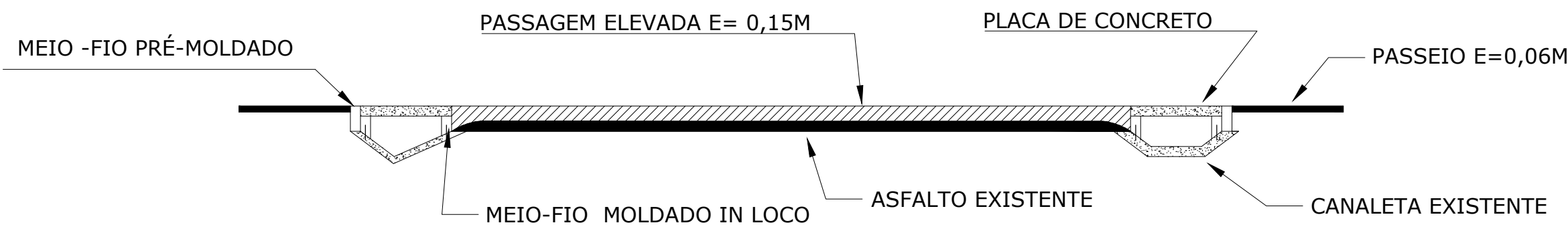
CORTE - AA ESC. 1:50
