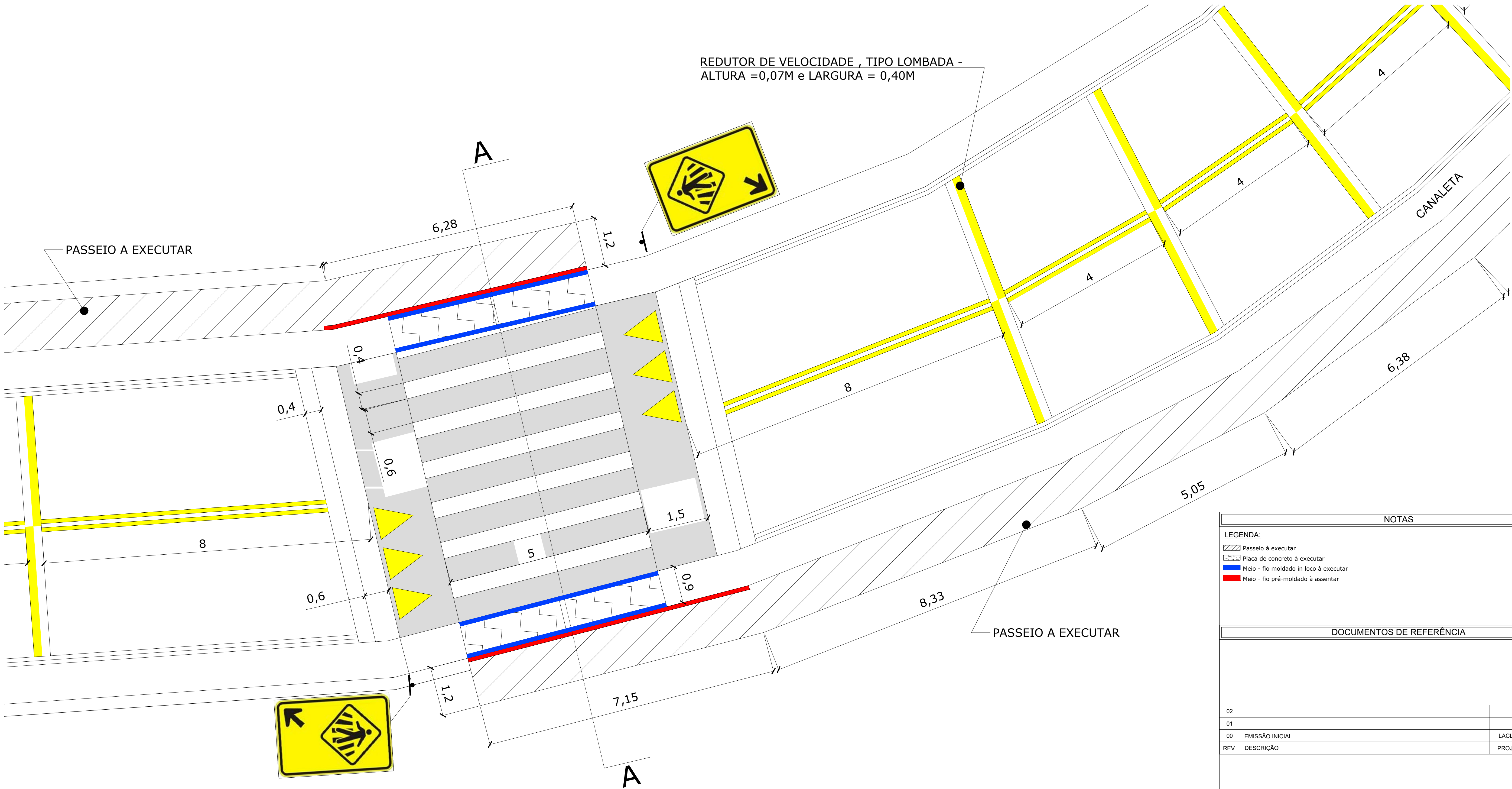
DETALHE 4 ESC. 1:50
