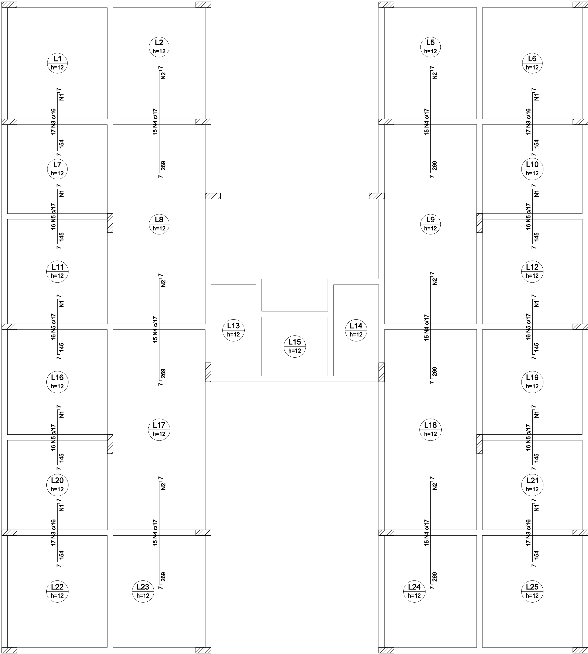
Armação negativa da 1ª laje (Eixo Y) escala 1:50
