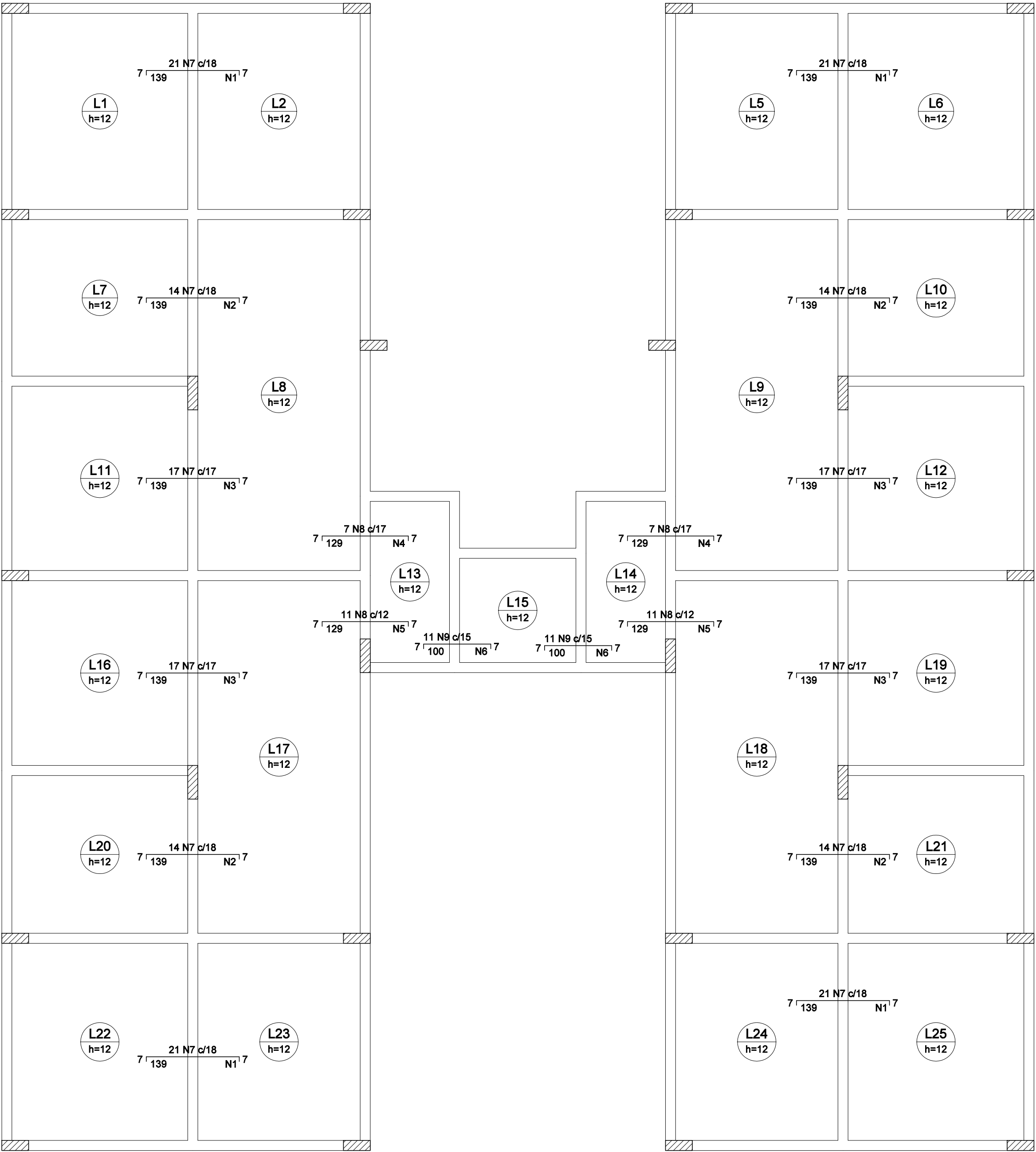
Armação negativa da 1ª laje (Eixo X) escala 1:50
