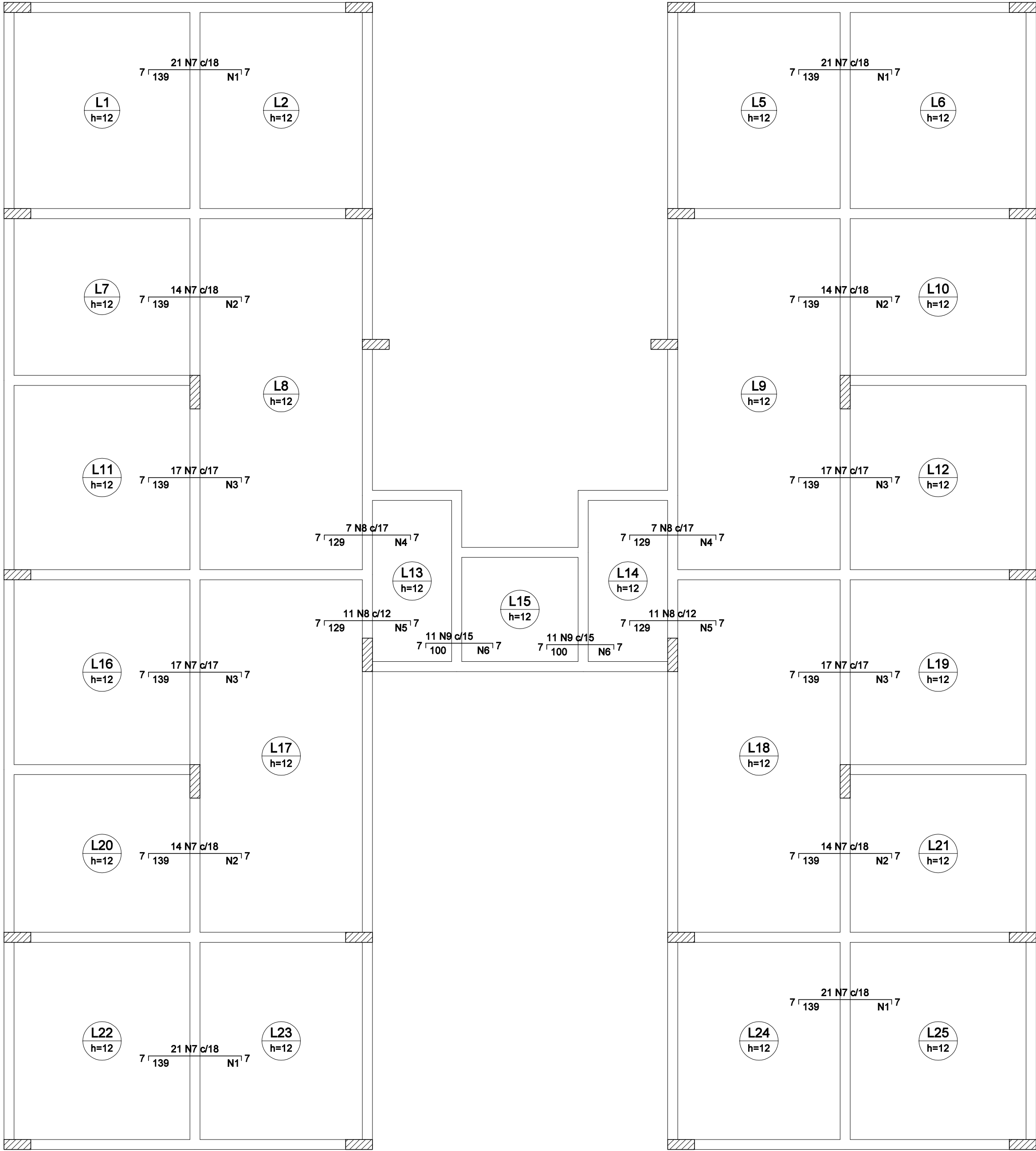
Armação negativa da 2ª e 3ª laje (Eixo X) escala 1:50
