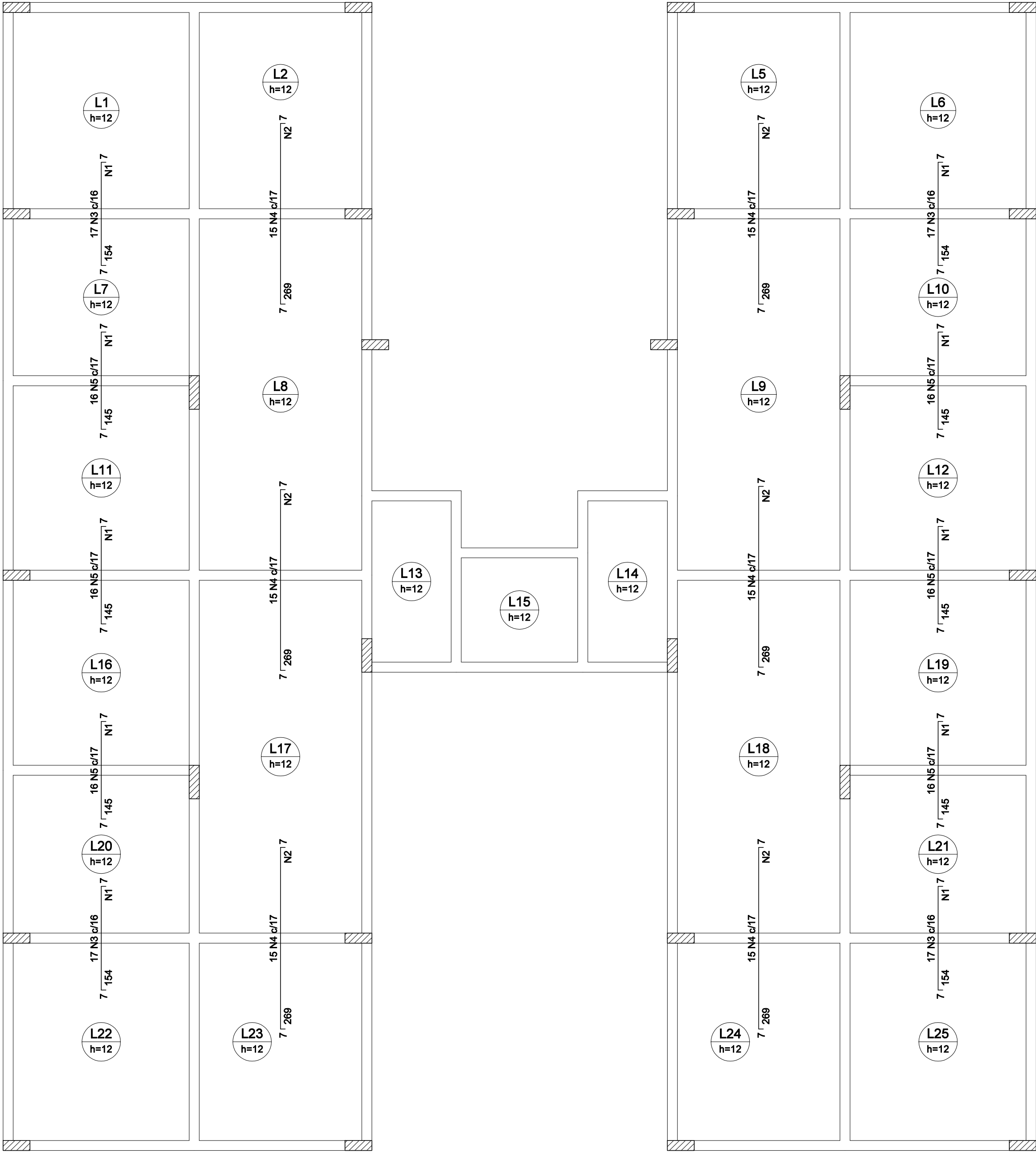
Armação negativa da 2ª e 3ª laje (Eixo Y) escala 1:50
